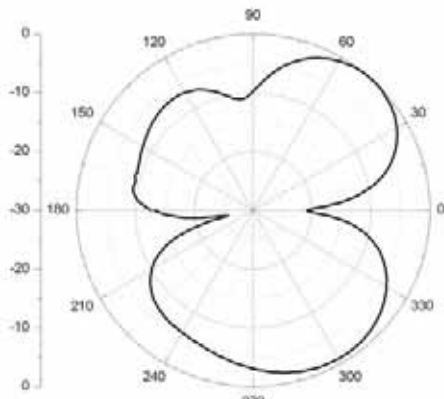
H-Plane
