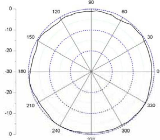
E-Plane
