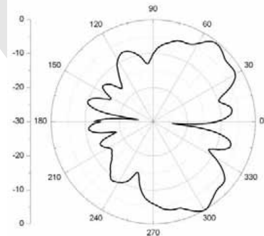
H-Plane
