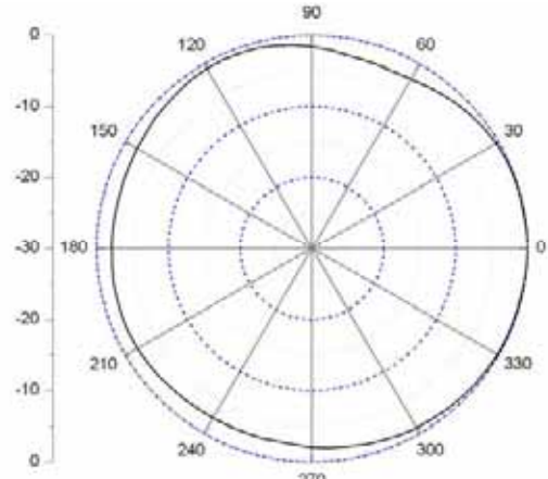
E-Plane
